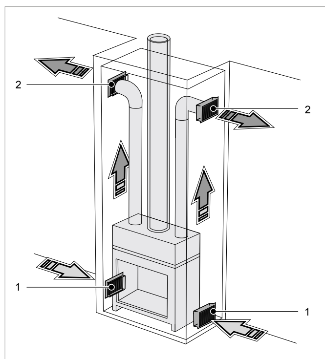
Figuur 17: Ombouw haard met convectiemantel
