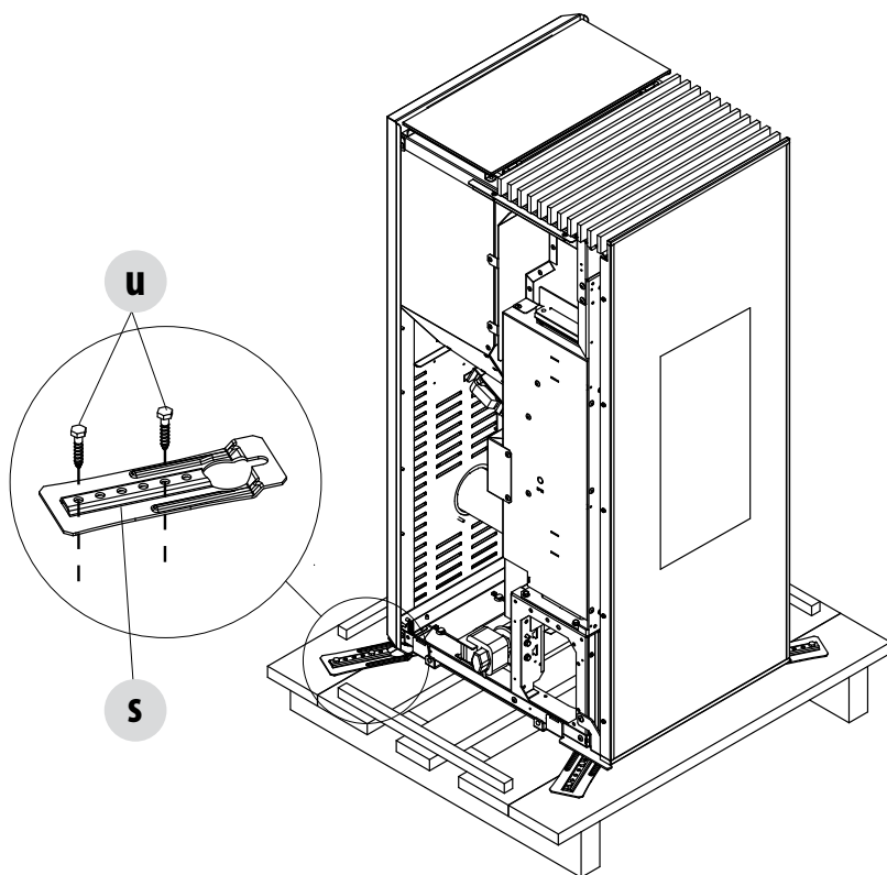
VERWIJDERING BEVESTIGINGSBEUGELS
