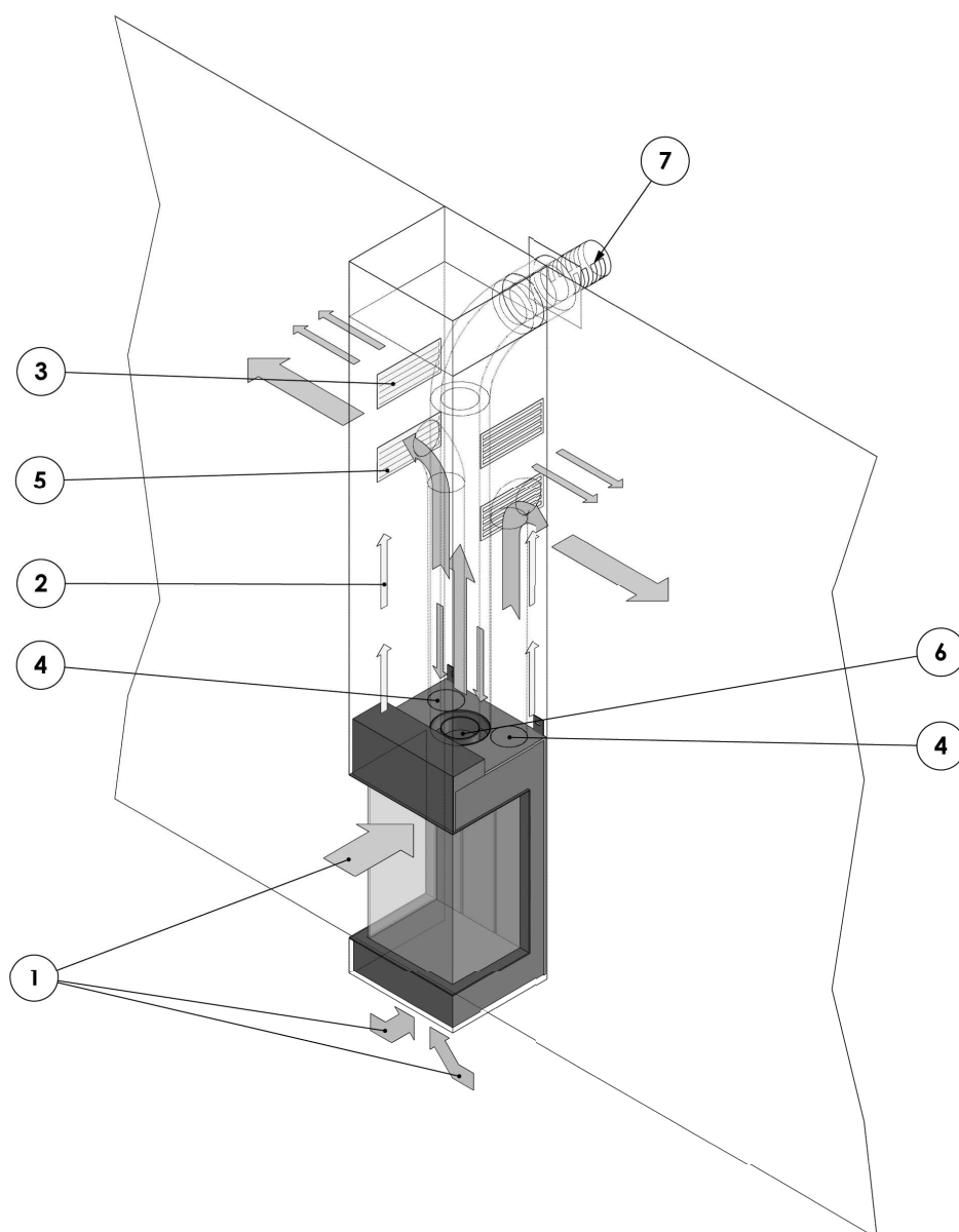
Figuur 18: HANG-HAARD: Toestel met geventileerde koof Horizontale uitmondung van de rookgasafvoer/verbrandingslucht- toevoer via de muur. Voorzien van de opties/accessoires: • convectiepakket (= convectiemantel en 1x convectieset)
