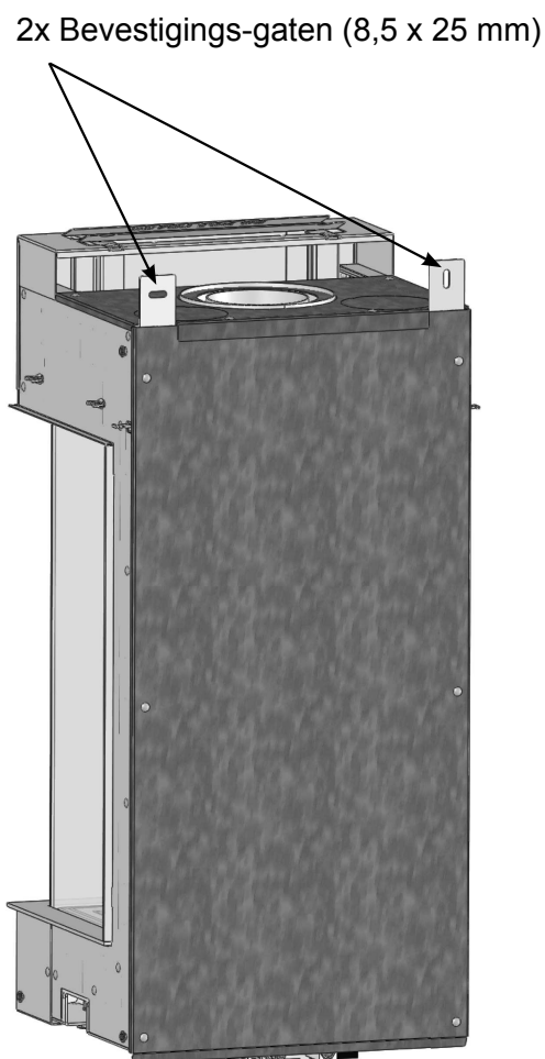
Figuur 21: Bevestigingsgaten (2x) Achterzijde Hang-Haard
