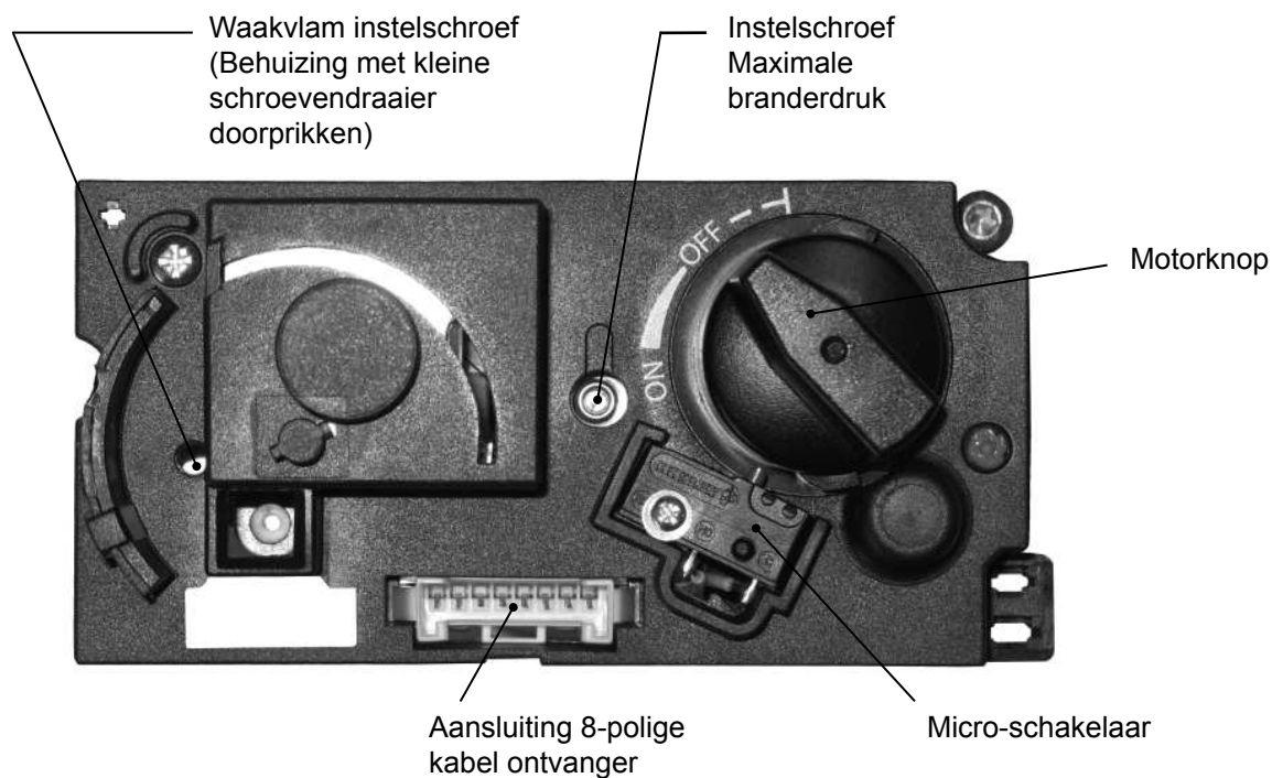
Figuur 24: Gasregelblok - Voorzijde
