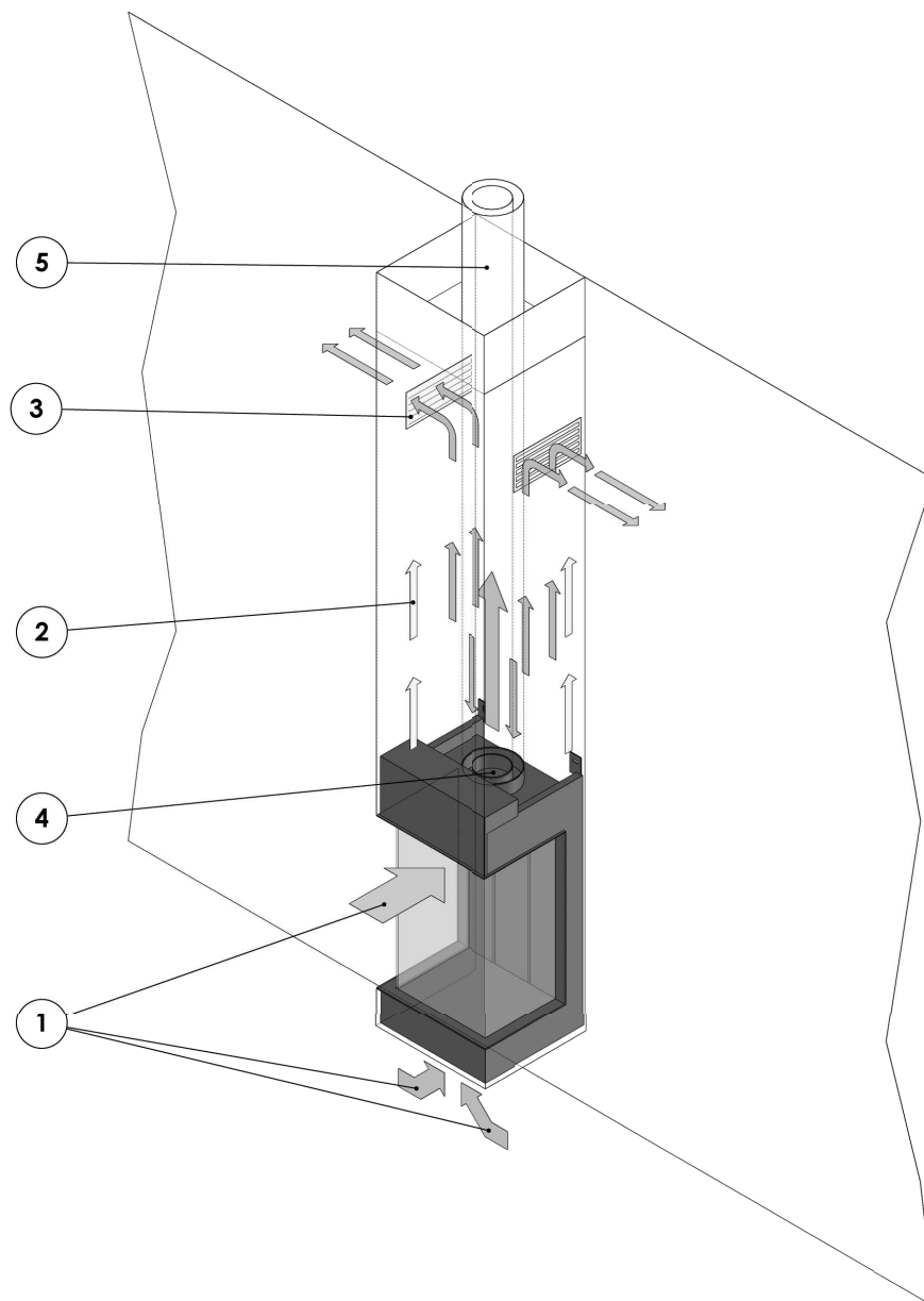
Figuur 19: HANG-HAARD: Toestel met geventileerde koof Verticale uitmonding van de rookgasafvoer/verbrandingslucht- toevoer via het dak. Toepassing zonder convectiepakket
