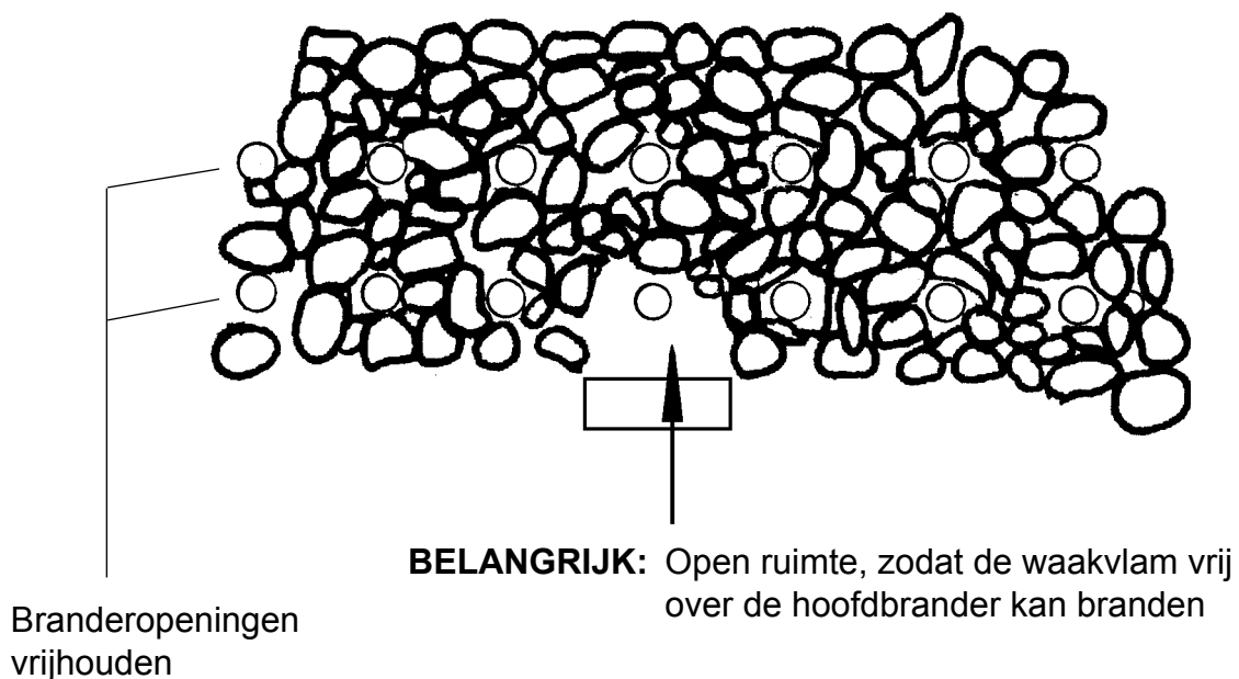
Figuur 30: Marmersplit-set aardgas- en propaan/butaan-brander
