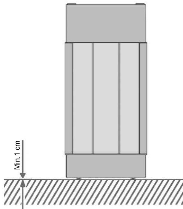
Figuur 15: Minimaal 1 cm ruimte tussen onderzijde toestel en vloer
