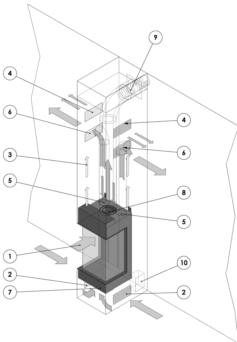
Figuur 16: INBOUW-HAARD: Toestel ingebouwd in geventileerde schouw Horizontale uitmonding van de rookgasafvoer/verbrandingslucht- toevoer via de muur. Voorzien van de opties/accessoires: • convectiepakket (= convectiemantel en 1x convectieset)
