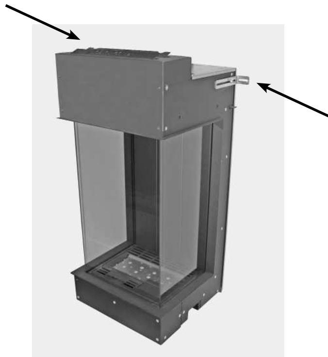
Figuur 20: Bevestigingsbeugel (2x)
