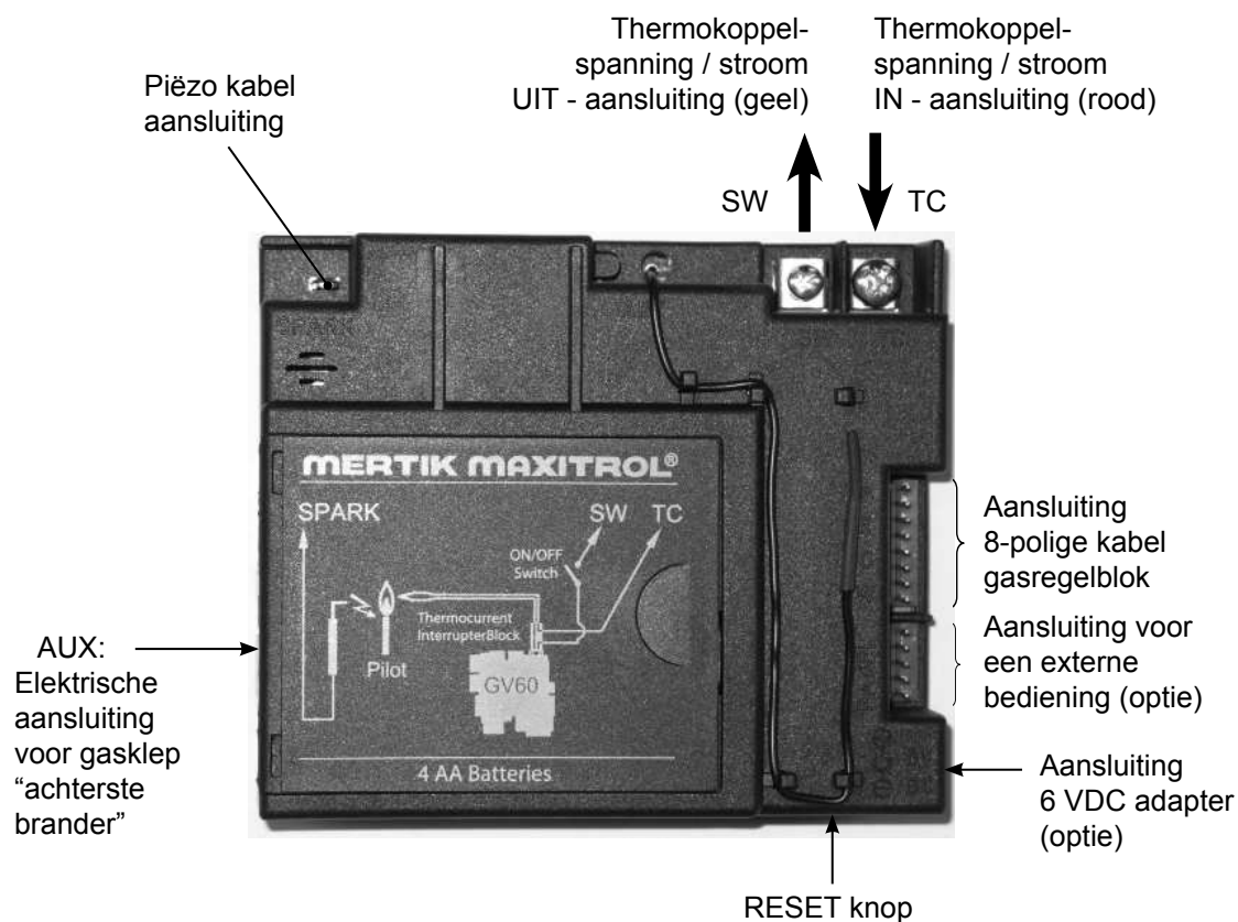
Figuur 26: Ontvanger - Bovenzijde
