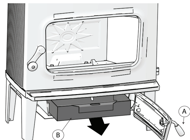
Afb. 14 Aslade
