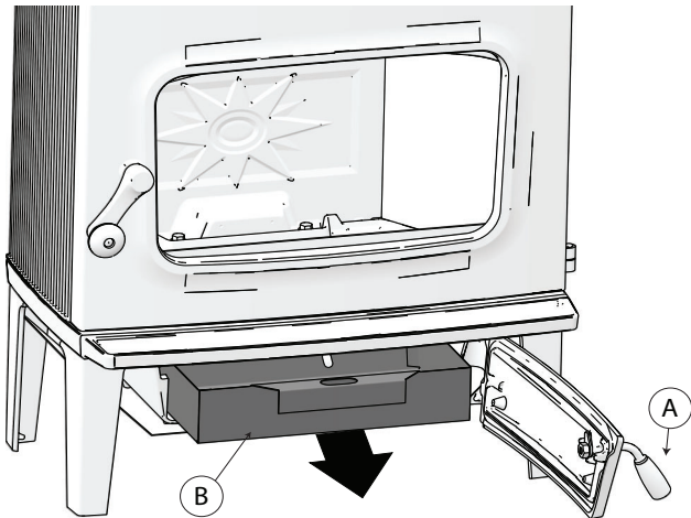
Abb. 14 Aschenkasten
