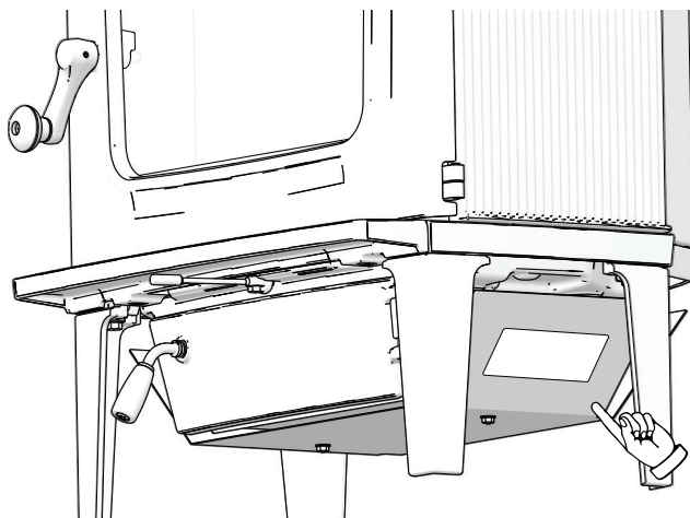
Abb. 9 Zulassungsetikett
