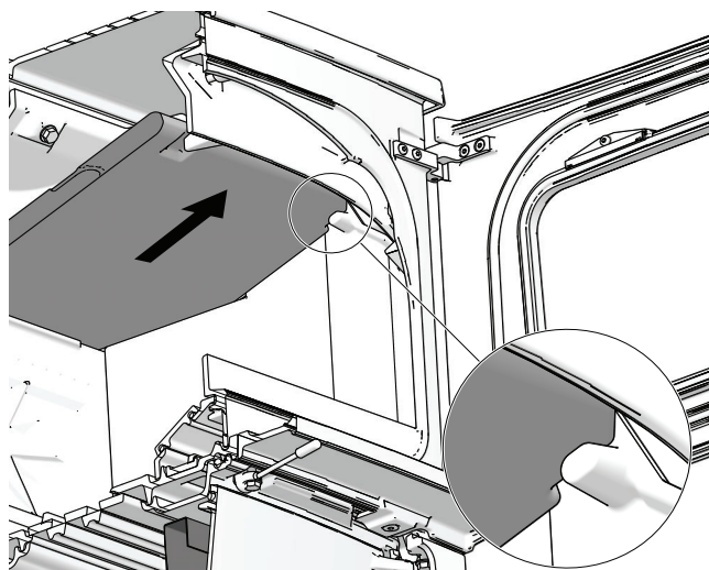
Abb. 16a Lösen der Leitbleche
