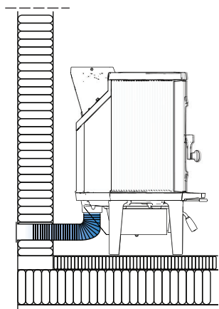
Rys.7a Podłączenie wykonane przez ścianę zewnętrzną
