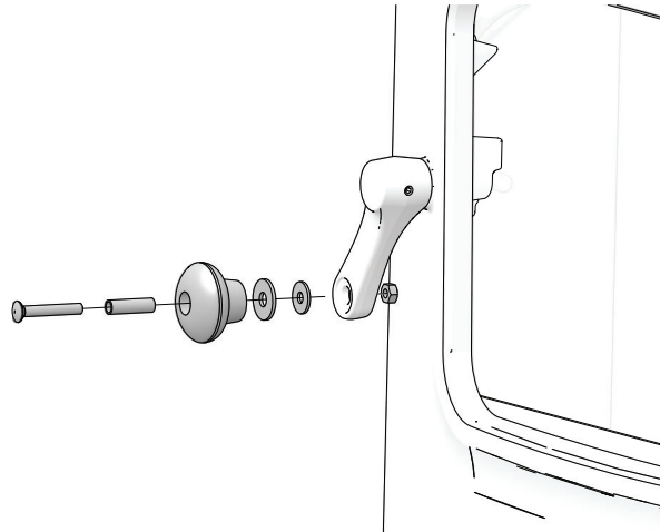
Afb. 3 Monteer de hendel voor de deur.
