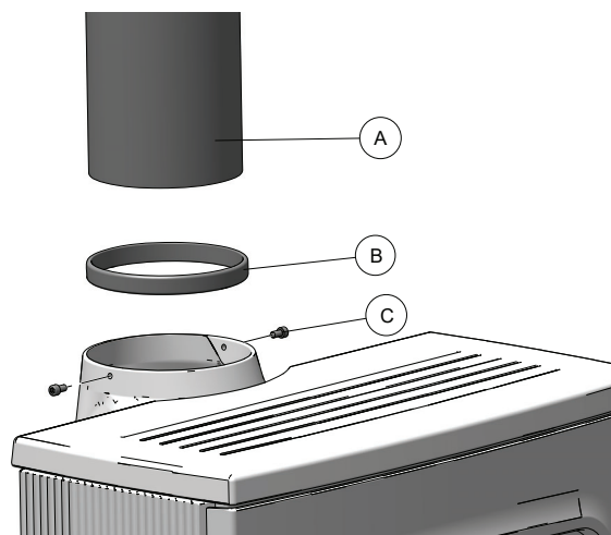
Abb. 6 Montage des Rauchgasrohrs
