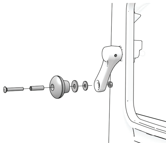
Abb. 3 Montage des Türgriffs
