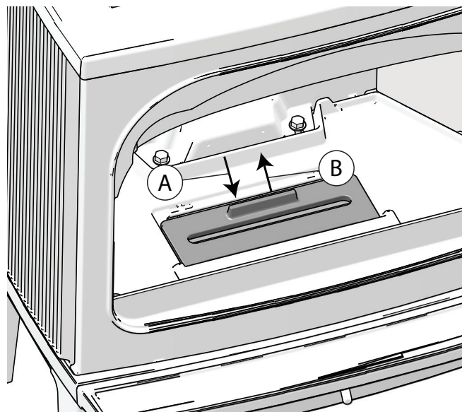
Abb. 13 Aschenrost
