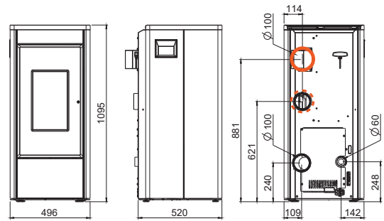
PRIMO MULTIAIR 8 kW
