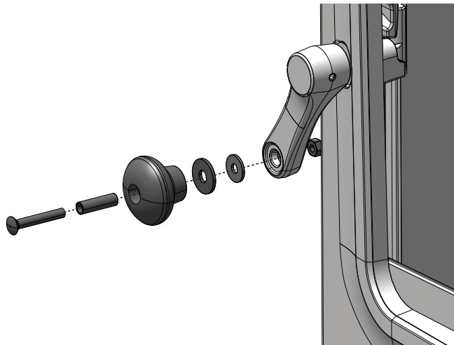
Fig. 3b Installazione della maniglia dello sportello (F 205 V2 - Modern)
