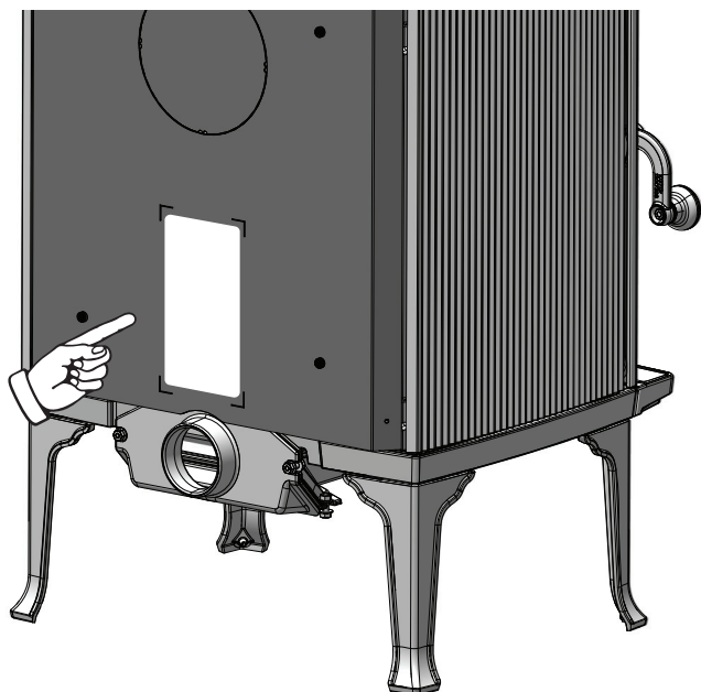
Bild 10 – Zulassungsetikett
