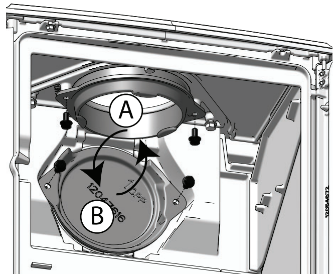
Afb. 4a Wisselen van boventuitlaat naar achteruitlaat
