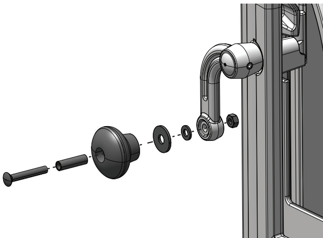
Afb. 3a Installatie van de deurehendel (F 200 V2 - klassiek)
