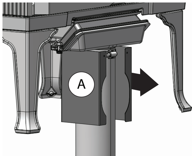
Fig. 9 Montering av deksel for friskluft (tillvæl - 50061978)
