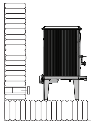
Kuva 7 Raitisilmaliitännän asennus
