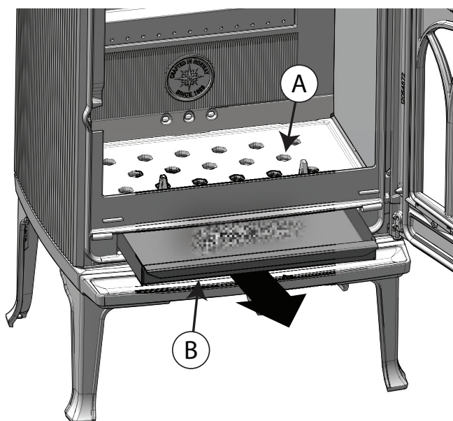
Afb. 14 Asrooster
