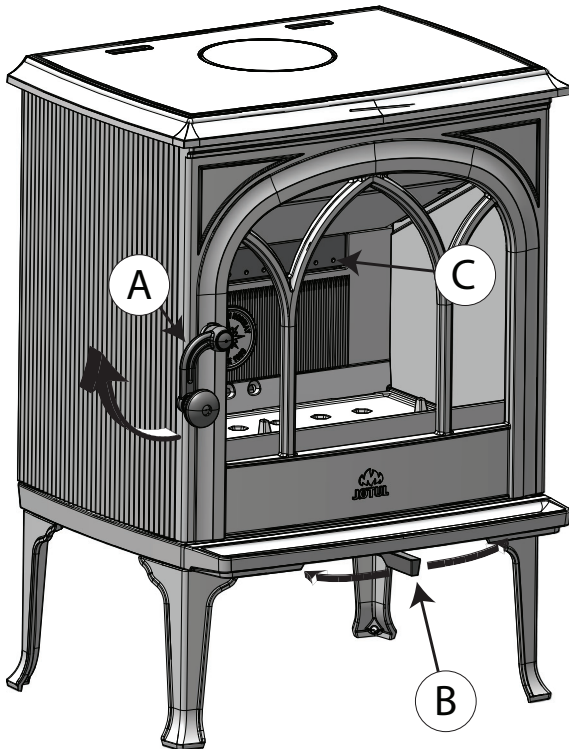
Afb. 11 Gebruiksopties van Jøtul F 200 V2/F 205 V2
