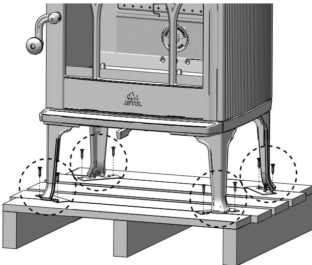
Afb. 2 Losmaken van pallet
