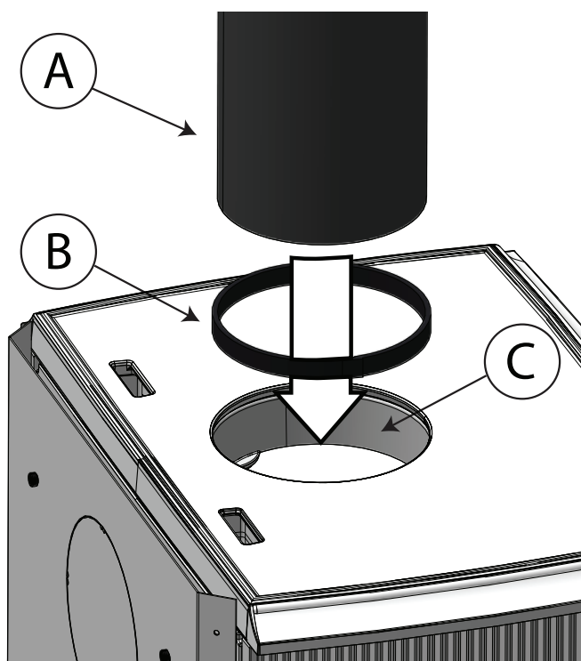
Fig. 5 Montere røykrør
