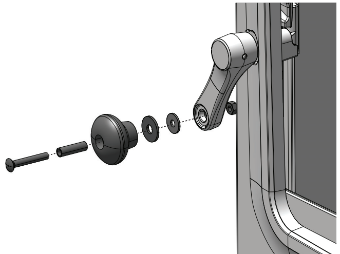
Afb. 3b Installatie van de deurehendel (F 205 V2 - modern)
