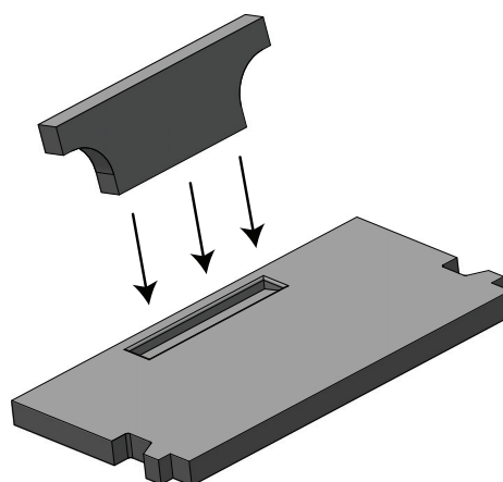
Bild 18 – Austausch des oberen Auslassleitbleches
